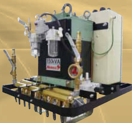
NTR05/NTR07+ PH5S (150kVA, 180kVA, 200kVA) 交流ポータブルトランス・タイマー一体式 Combine Type Transformer with Controller 交流手提式変圧器・計器一体式
