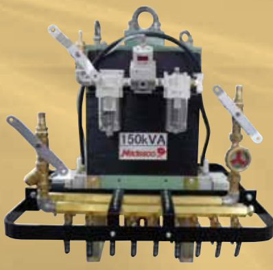
NTR05/NTR07 (150kVA, 180kVA, 200kVA) 交流ポータブルトランス・タイマ分体式 Separate Type Transformer 交流手提式変圧器・計器分体式
