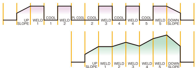
多段通電 Multiple Pulse Welds 多阶梯的输电
